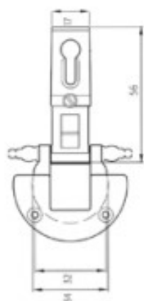
Scodellino totalmente incassato
