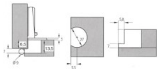
Scodellino parzialmente incassato
