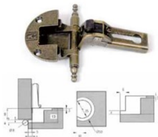
Scodellino totalmente incassato
